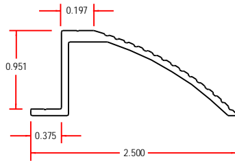
INSIDE JAMB SILL
